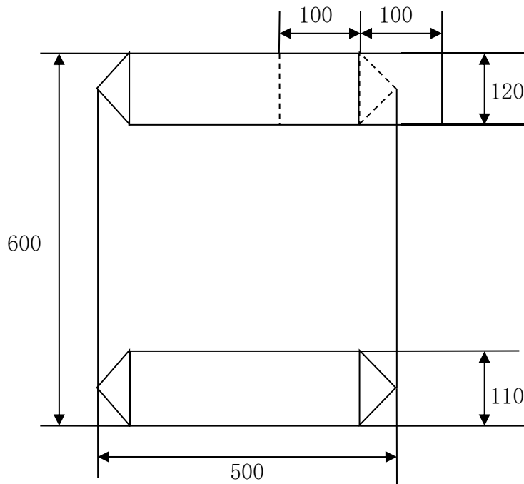
图6 阀口袋尺寸示意图
